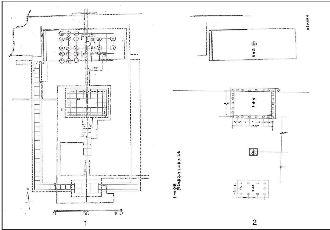
〈도면2〉 부여 정림사지 가람배치도(좌: 1971년 논문, 우: 梅原末治 考古資料)
