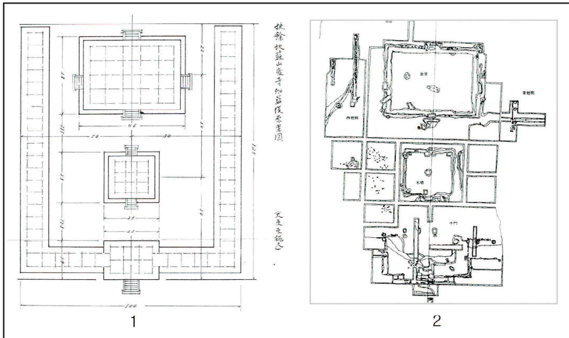
〈도면3〉 부여 부소산페사지 가람배치도(좌: 1976년 토론회, 우: 국립부여박물관)
